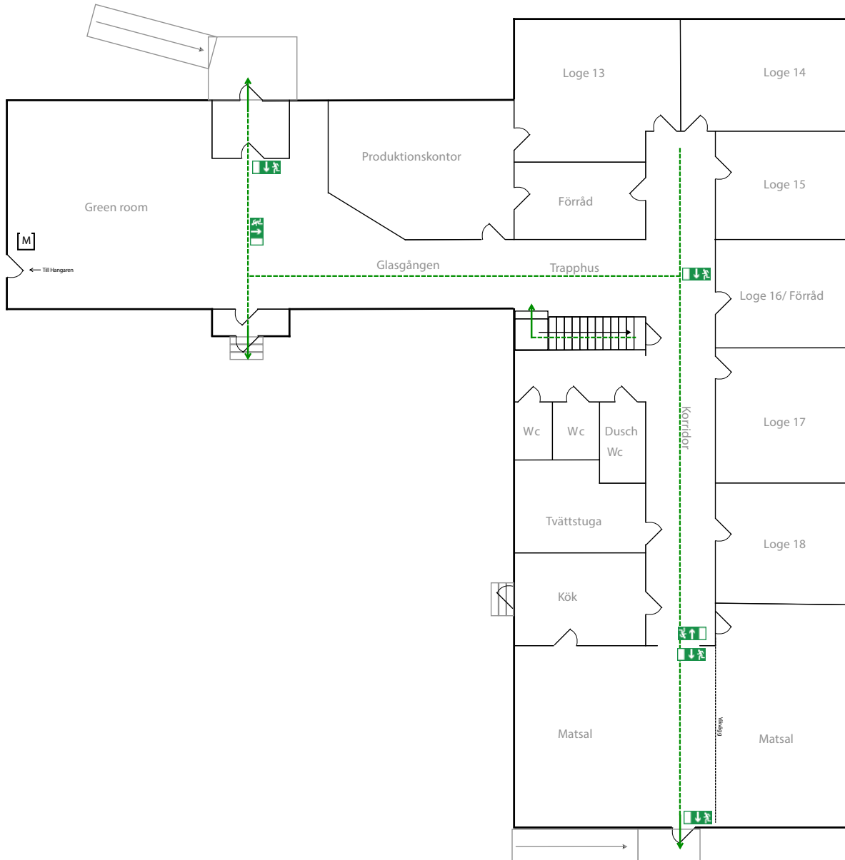
Nedre plan
